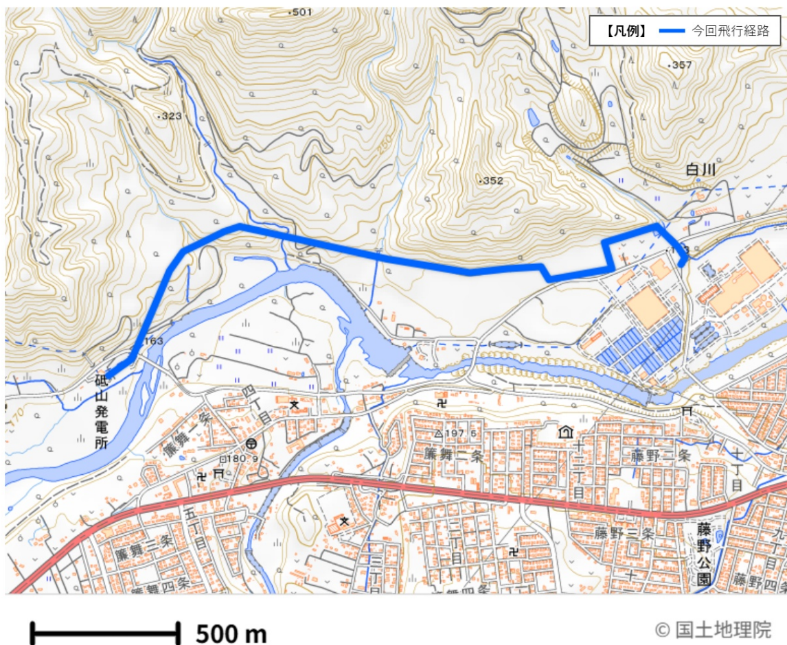
飛行経路図
